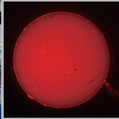
太陽 (H \alpha 譜線)
